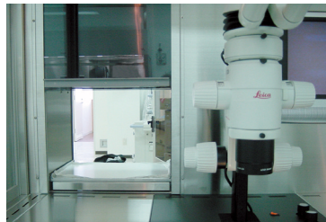
スライド式パスボックス取付け例
